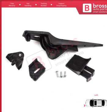
BHL556 Ford Fiesta B299 B409 B479 2013-2019 D2BZ13008L İçin Sol Ön Far Ayak Tamir Seti
