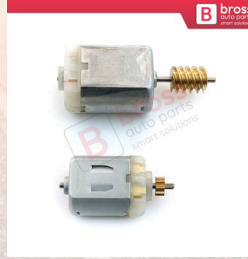
BGE661+BGE662 Ford Volvo Land Range Rover Jaguar Mazda İçin Kapı Kilit Motor Dişli Set
