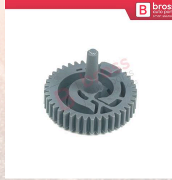
BGE642 Renault Clio Scenic Megane Twingo İçin Bagaj Kilit Dişlisi 8200102583
