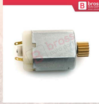
BGE665 Mercedes Axor Atego Actros İçin Kapı Kilit 24V Motor Dişli Seti
