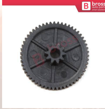
BGE607 Renault Clio İçin Klima Motor Klepe Tamir Dişlisi Diş Sayısı: 56/10
